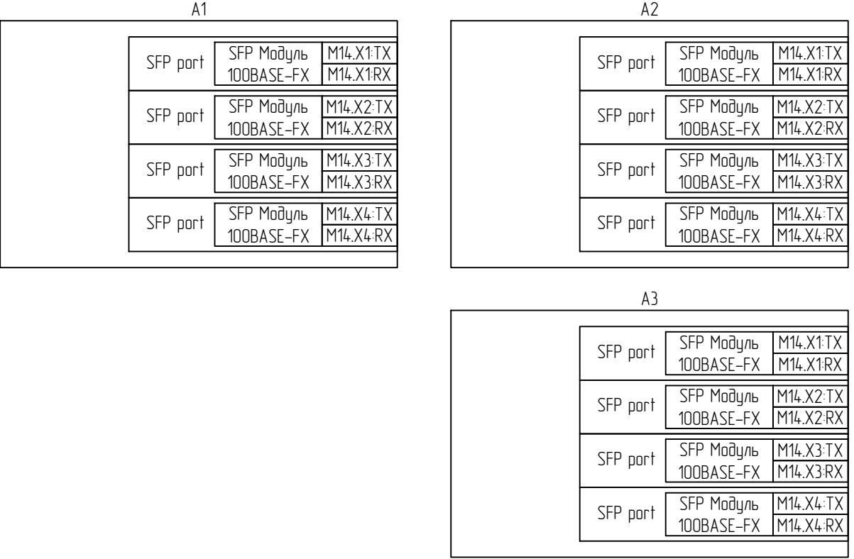
Цепи портов связи терминала
