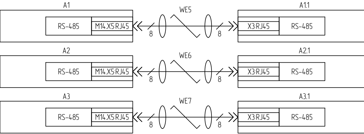
Цепи портов связи терминала с ИЧМ
