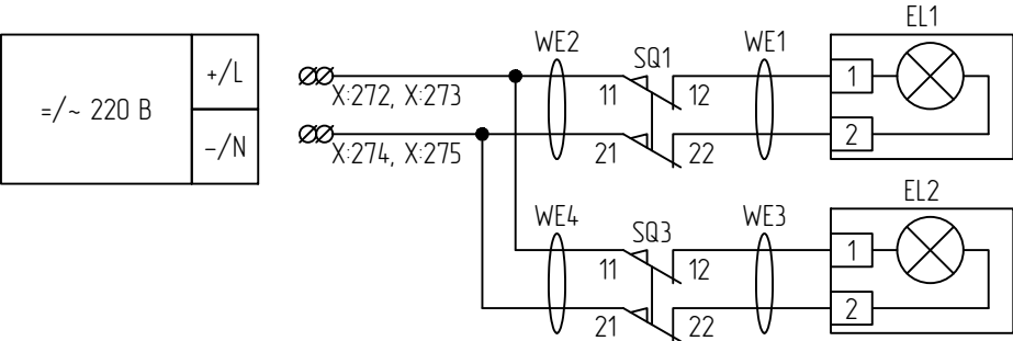
Цепи освещения шкафа
